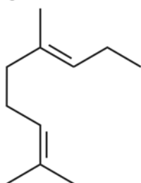
geraniol
