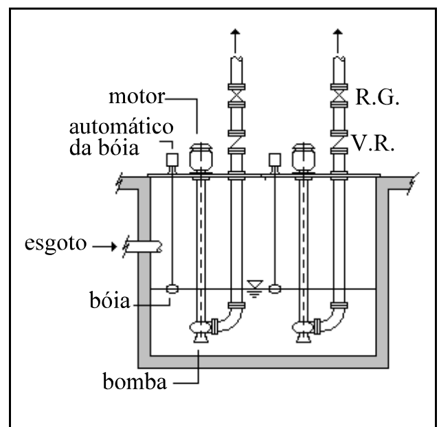
A. J. Macintyre. Instalações hidráulicas prediais e industriais, LTC, 1996 (com adaptações).
