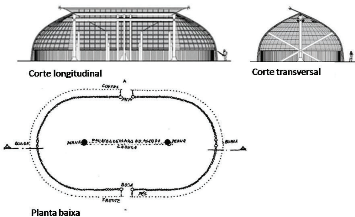
Figuras 10, 11 e 12: Cortes e planta da Casa Xinguana
